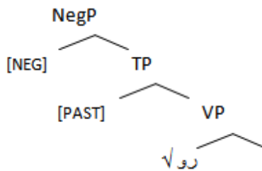
نمودار (۳). ترتیب سلسله‌مراتب نحوی گره‌های نفی، زمان و فعل اصلی در فعل «نفت»
